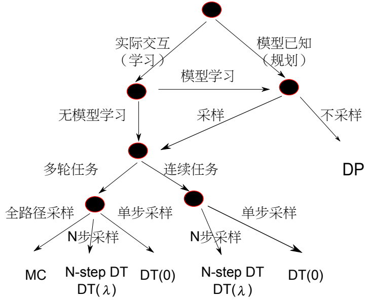
Fig. 10.13 TD、MC、DP三种学习方法的应用场景。
