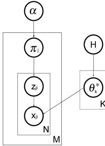
Fig. 8.6 LDA主题模型的有向图模型表示。对第 j 篇文档由狄利克雷分布生成一个主题分布概率 \pi_j ，对该文档中的每个词，由 \pi_j 生成一个主题变量 z_i ，基于该主题变量，由 Multi(\theta_{z_{ji}}) 生成词 x_{ji} 。主题 \theta_k^* 由一个以 H 为基础变量的狄利克雷分布生成。
