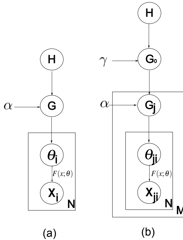
Fig. 8.14 基于DP(左)与HDP(右)的数据生成模型。 F(x; \theta) 为数据分布概率。在HDP中，每个场景 j 由共享的 DP(\gamma, H) 中得到 G_0 ，再由 DP(\alpha, G_0) 得到不同场景下的概率 G_j 。由 G_j 可以得到每个数据样本对应的模型参数 \theta_{ji} ，进而生成数据 x_{ji} 。
