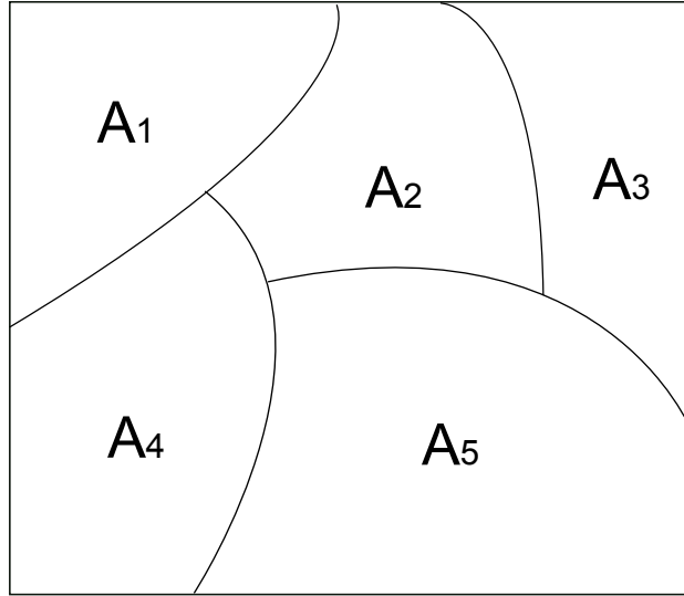
Fig. 8.9 狄利克雷过程是无限维空间 X 上随机分布，该分布满足如下概率一致性：对 X 的任何划分，其累积概率符合狄利克雷分布。图中 A_1 - A_5 是 X 一个划分， G(A_i) = \int_{x \in A_i} G(x) dx 。 G(A_1, A_2, A_3, A_4, A_5) = \text{Dir}(\alpha H(A_1), \alpha H(A_2), \alpha H(A_3), \alpha H(A_4), \alpha H(A_5)) 。
